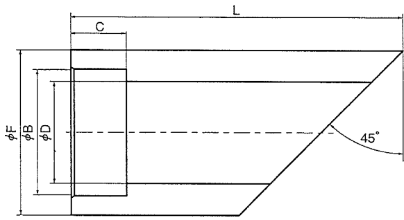
SW 45°カットボス
