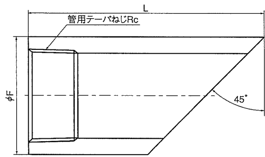
Rc (PT) 45°カットボス
