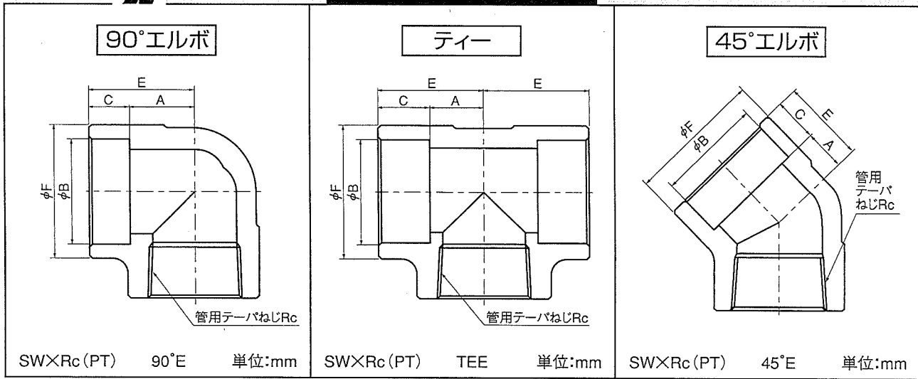
90°エルボ ティー 差込み式×ねじ込み式
