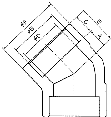
45°エルボ
